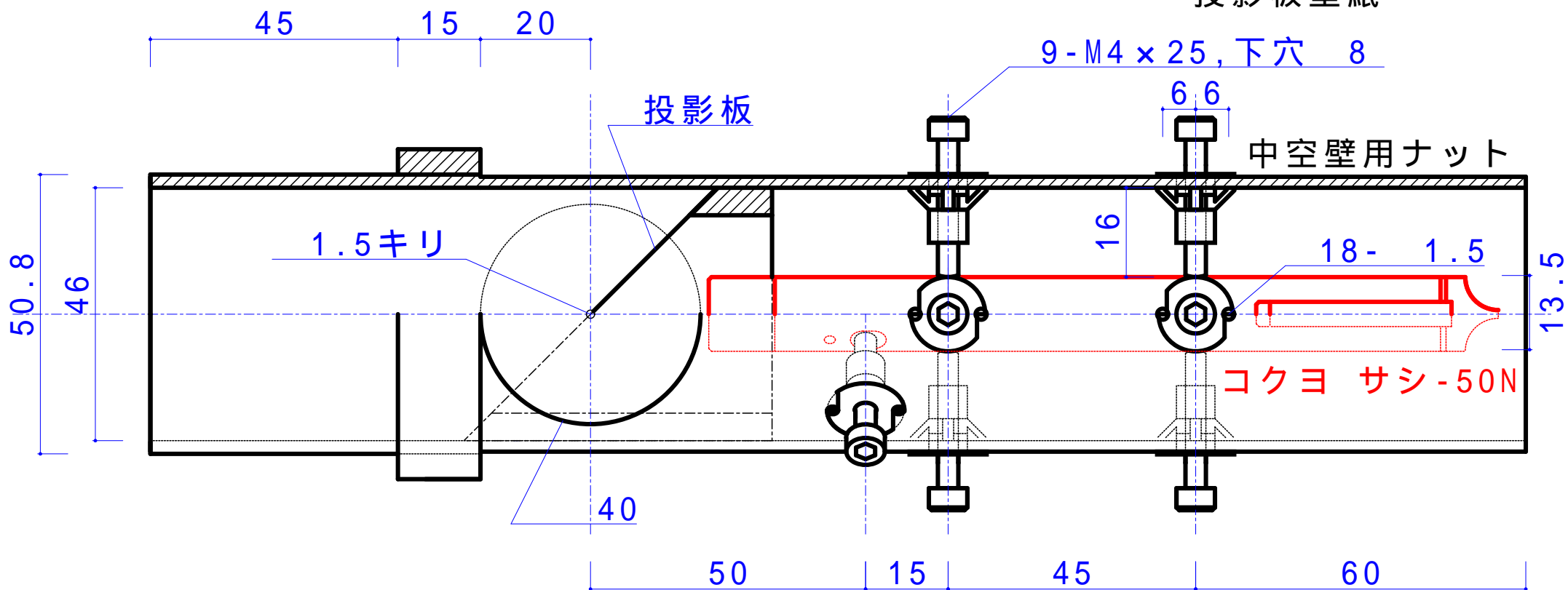
投影板型紙
